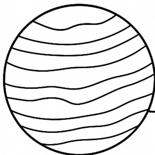
Jupiter
